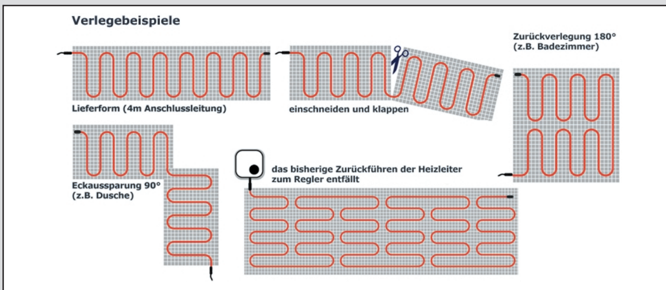
Verlegebeispiele
