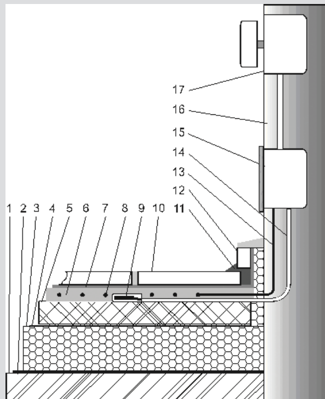
Funktionsaufbau Bodentemperierung
